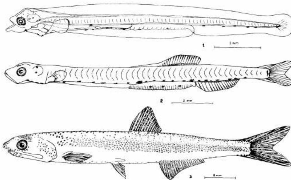
Final del desarrollo larval de la anchoíta ( Engraulis anchoita ). 1. Larva de 6 mm; 2. Larva de 13,5 mm; 3. Juvenil de 44 mm. Tomado de Ciechowski (1963)
