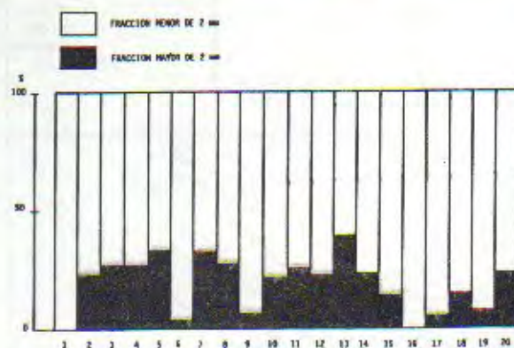
Fig. 3. Porcentaje en peso de la fracción sedimentológica mayor y menor de 2 mm en el área de estudio.
