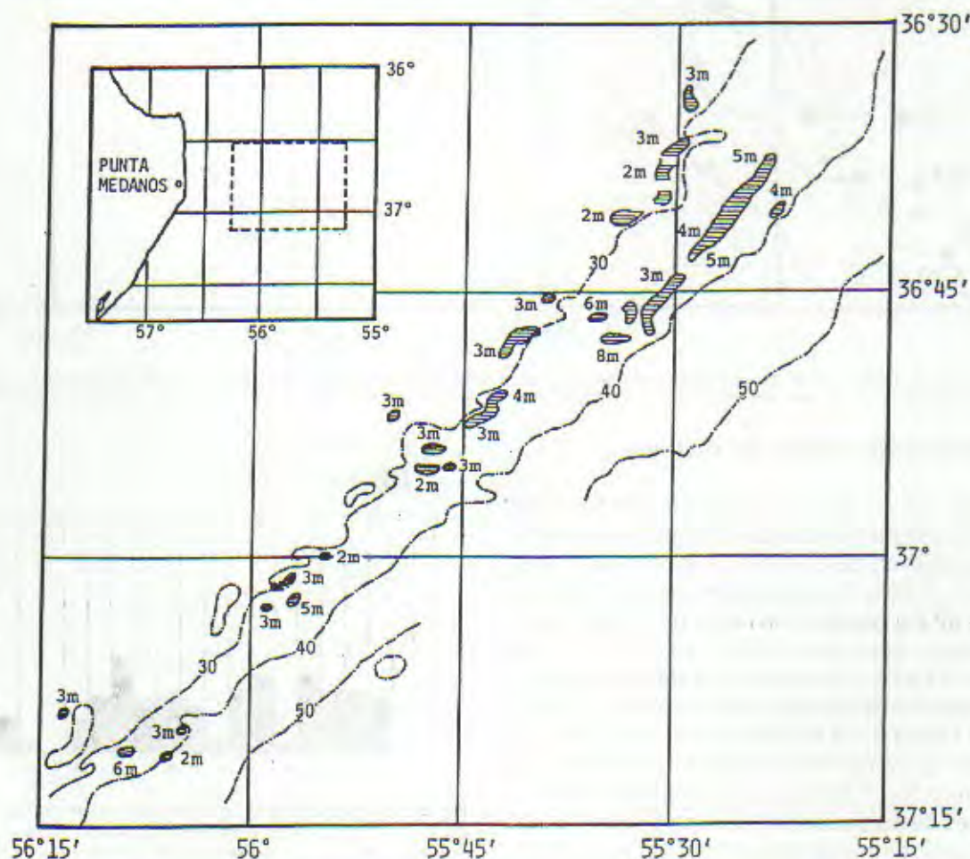
Fig. 1. Ubicación de los afloramientos y altura de los mismos con respecto al fondo (en metros) en el banco de pesca del besugo (Provincia de Buenos Aires, Argentina).
