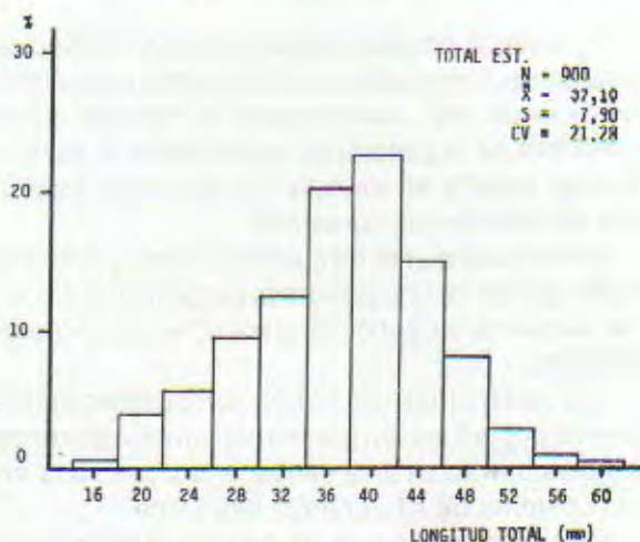
Fig. 10. Distribución de frecuencia de tallas de Mytilus platensis en el conjunto de las estaciones de mayor abundancia.
