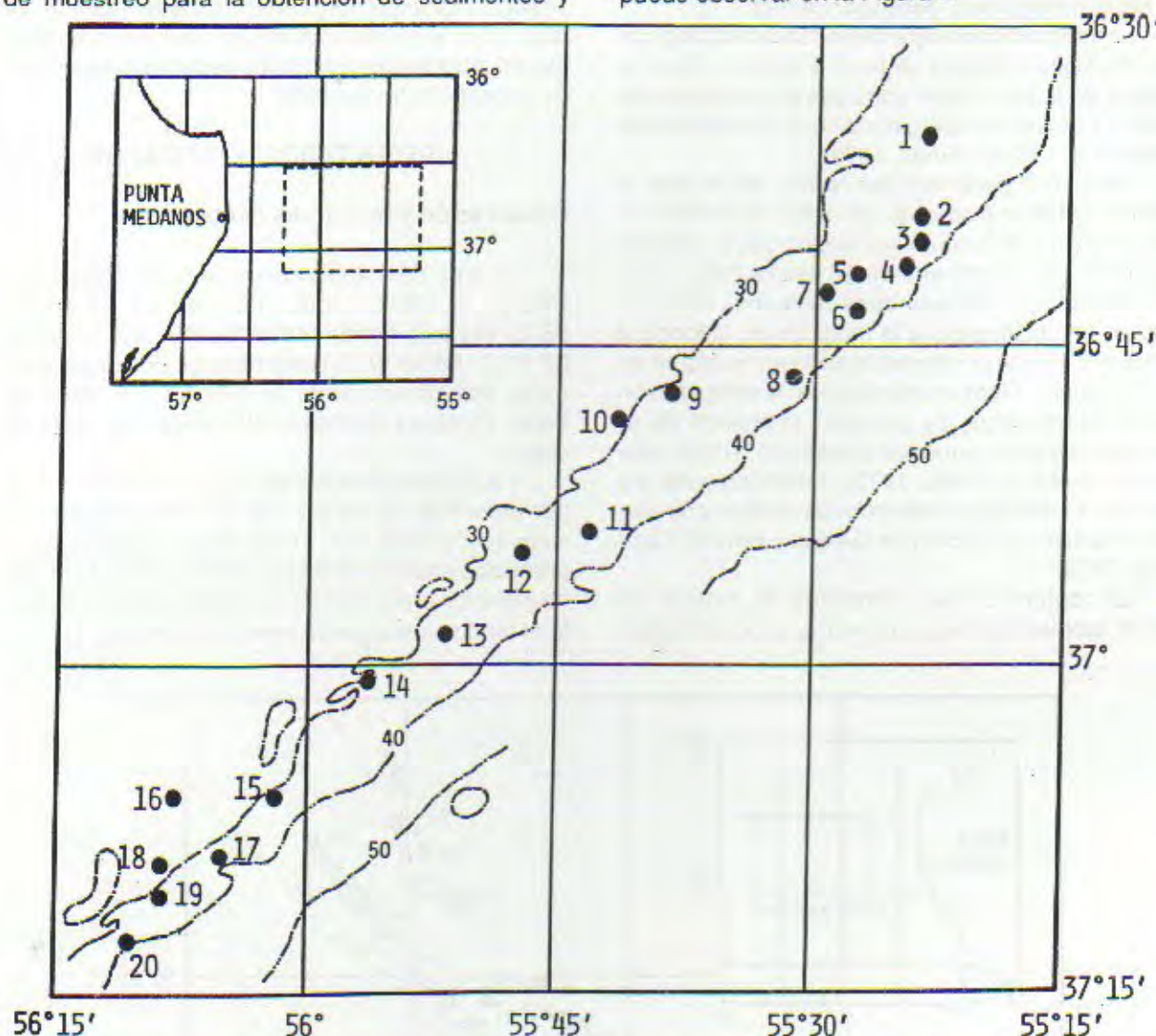
Fig. 2. Ubicación de las estaciones de muestreo en el área relevada (Provincia de Buenos Aires, Argentina).
